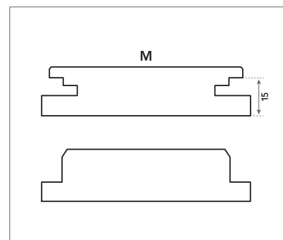
Szczegół krawędzi M: krawędź typu M pozwala tworzyć proste, wyraziste linie wzdłuż połączeń krawędzi nośnych i nienośnych.
